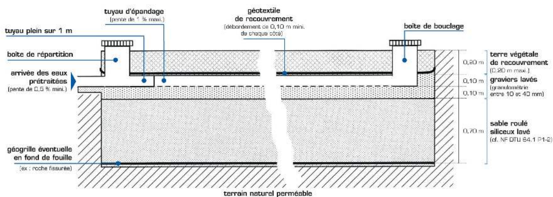
coupe longitudinale
